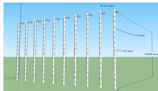
Gambar 4. Desain pipa pada Spray Aerator
