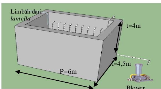
Gambar 2. Spray Aerator dilihat dari perspektif
