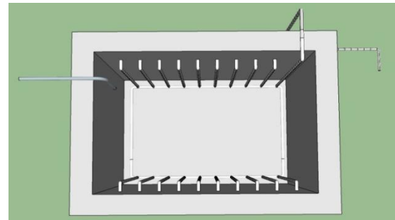
Gambar 3. Spray Aerator dilihat dari atas
