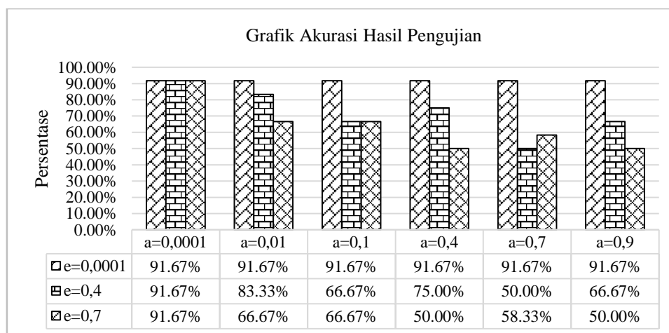
Gambar 4. Akurasi hasil pengujian dengan babarapa variasi parameter
